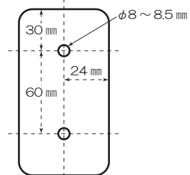
<助手席側フレーム 穴あけ位置参考寸法図>
