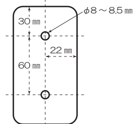
<運転席側フレーム 穴あけ位置参考寸法図>
