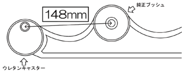
フロントリーディングアームのブッシュ取り付け寸法
