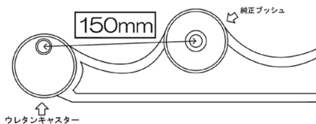
リアトレーリングアームのブッシュ取り付け寸法
